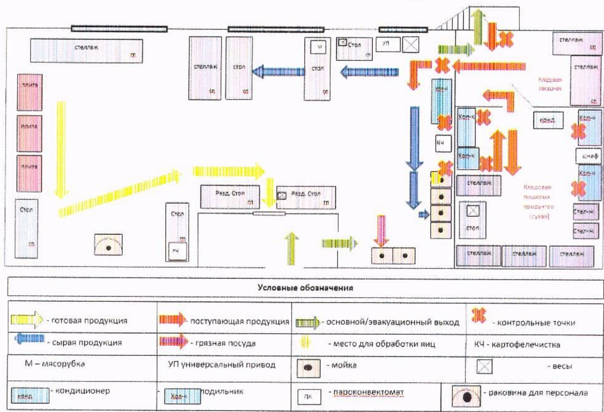
План-схема пищеблока в ГБДОУ детский сад №33 Московского района Санкт-Петербурга
