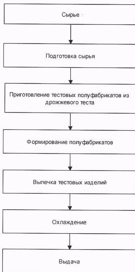
3.35 Блок-схема технологического процесса приготовления напитков
